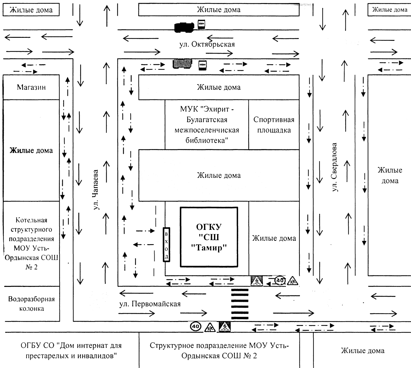
Схема организации дорожного движения в непосредственной близости от ОГКУ "СШ "Тамир" с размещением соответствующих технических средств организации дорожного движения, маршруты движения занимающихся и расположение парковочных мест
